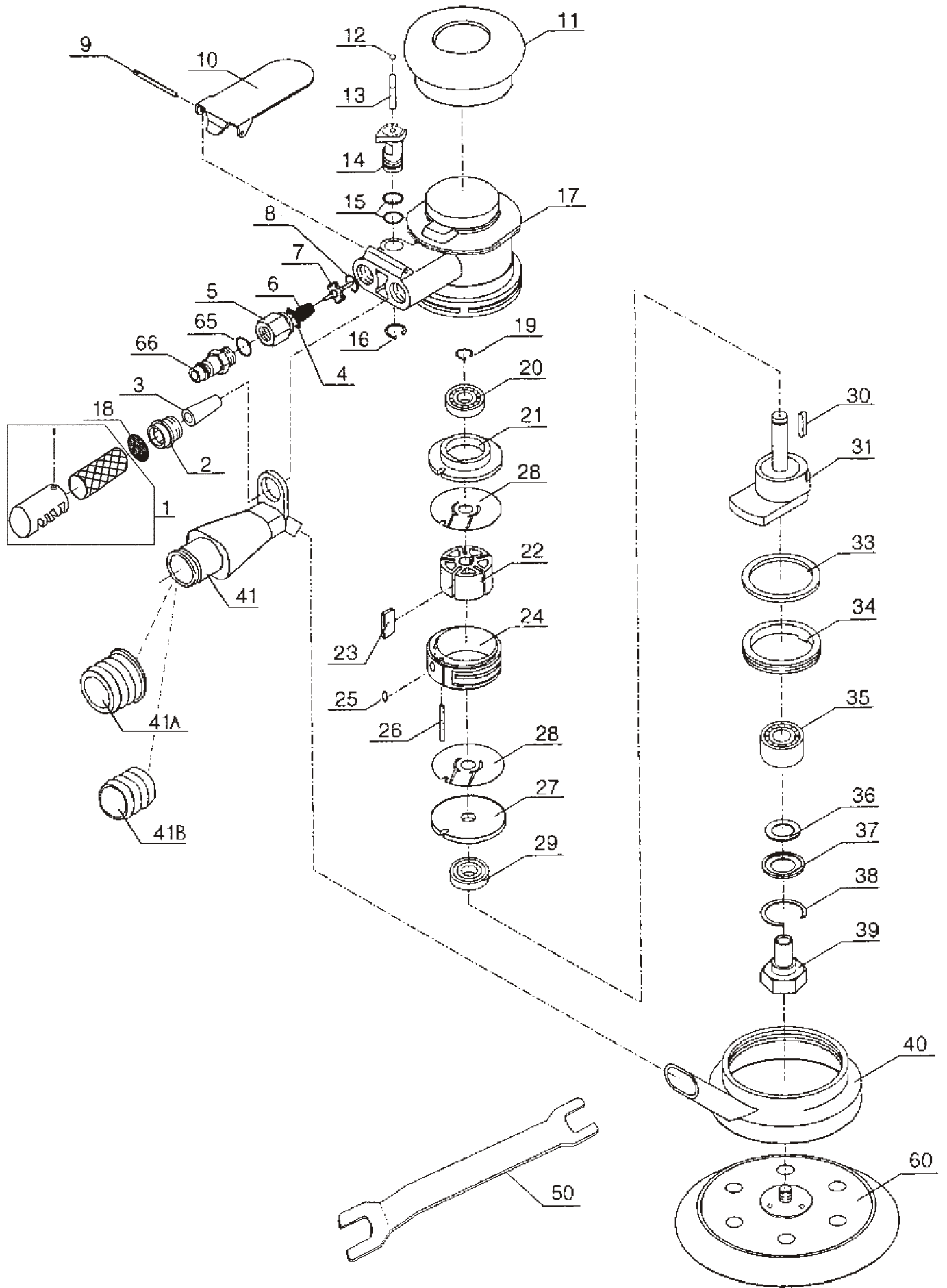
LEVIGATRICE PNEUMATICA CR 036 C
